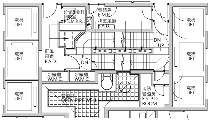
第3座(3A及3B) 22樓部分平面圖
