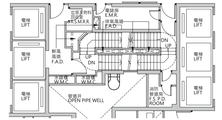
第3座(3A及3B) 50樓部分平面圖
