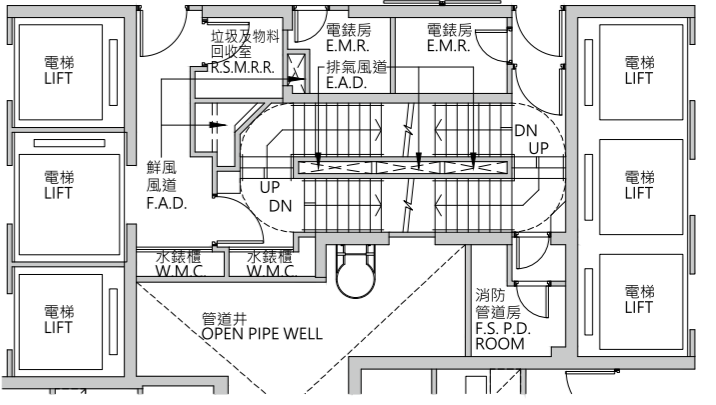
第3座(3A及3B) 47樓部分平面圖
