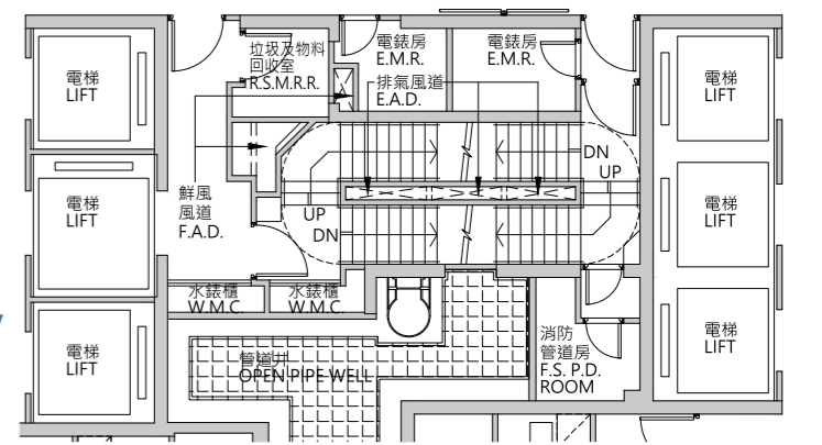
第3座(3A及3B) 66樓部分平面圖
