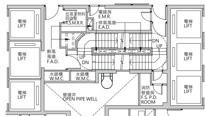
第3座(3A及3B) 20樓部分平面圖
