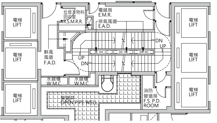
第3座(3A及3B) 48樓部分平面圖
